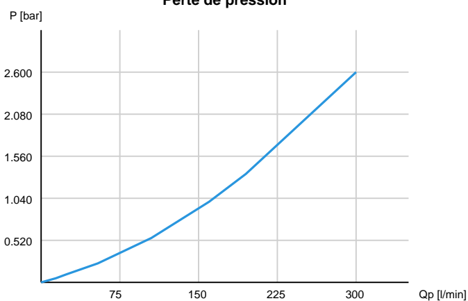
Perte de pression
