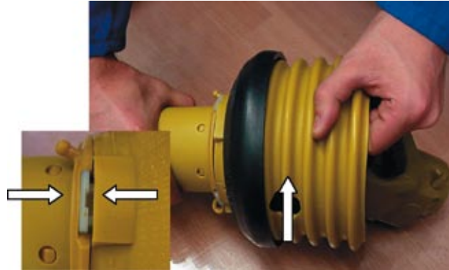
Trichter in Montageposition drehen.
