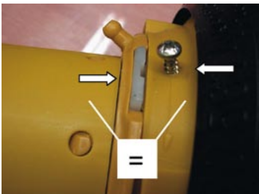
Arretierschraube mittig zur Gleitringkerbe eindrehen.
